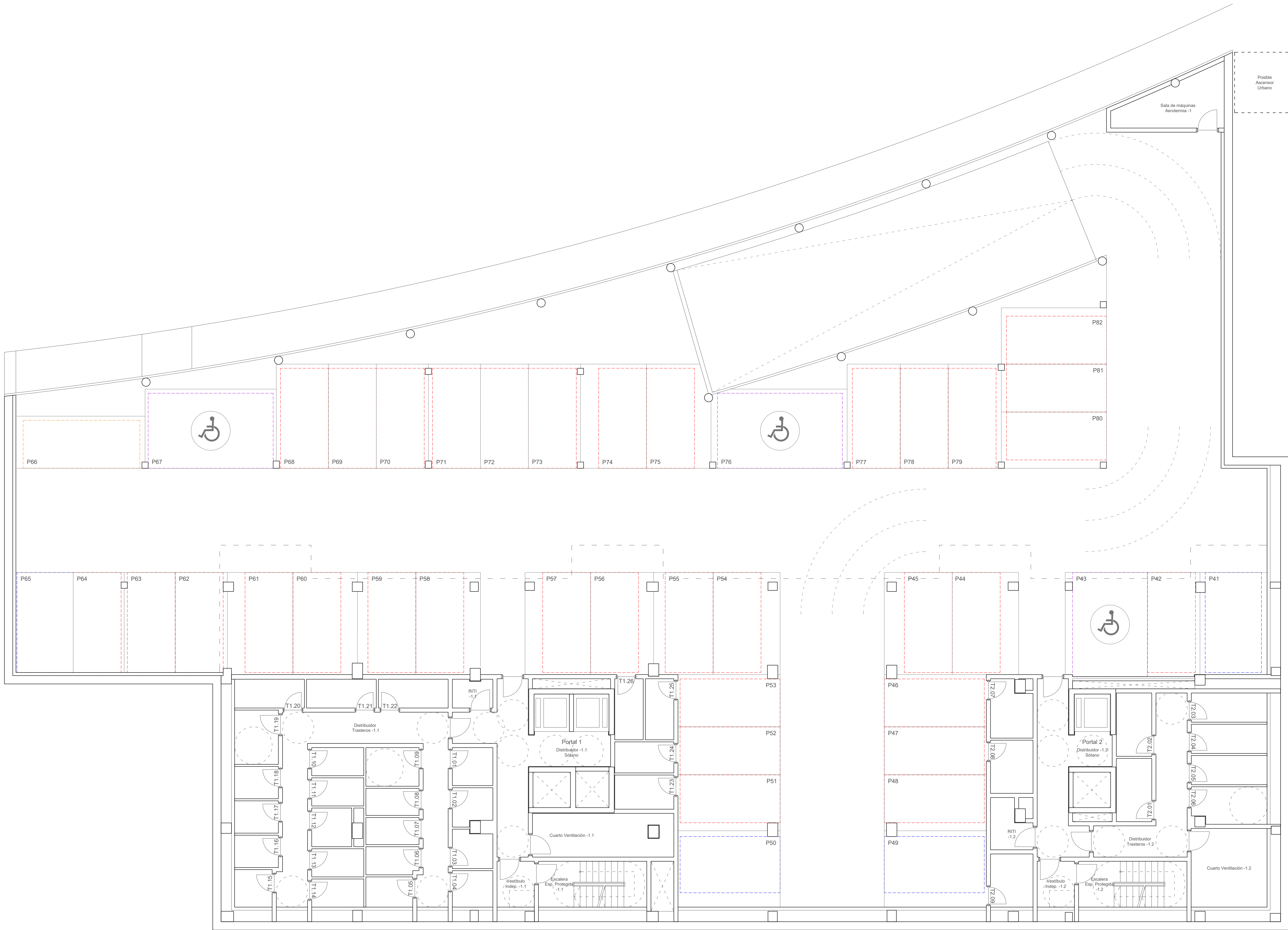
PLANTA SÓTANO -1 +21.00
