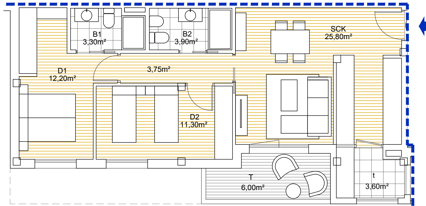
PLANTA PRIMERA
