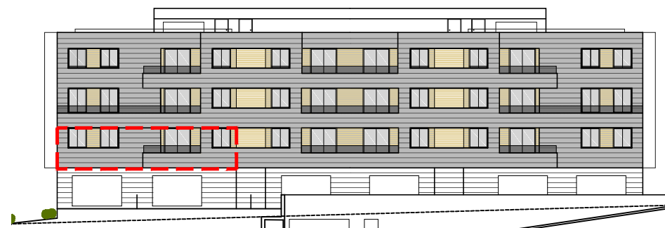
ALZADO TRASERO
