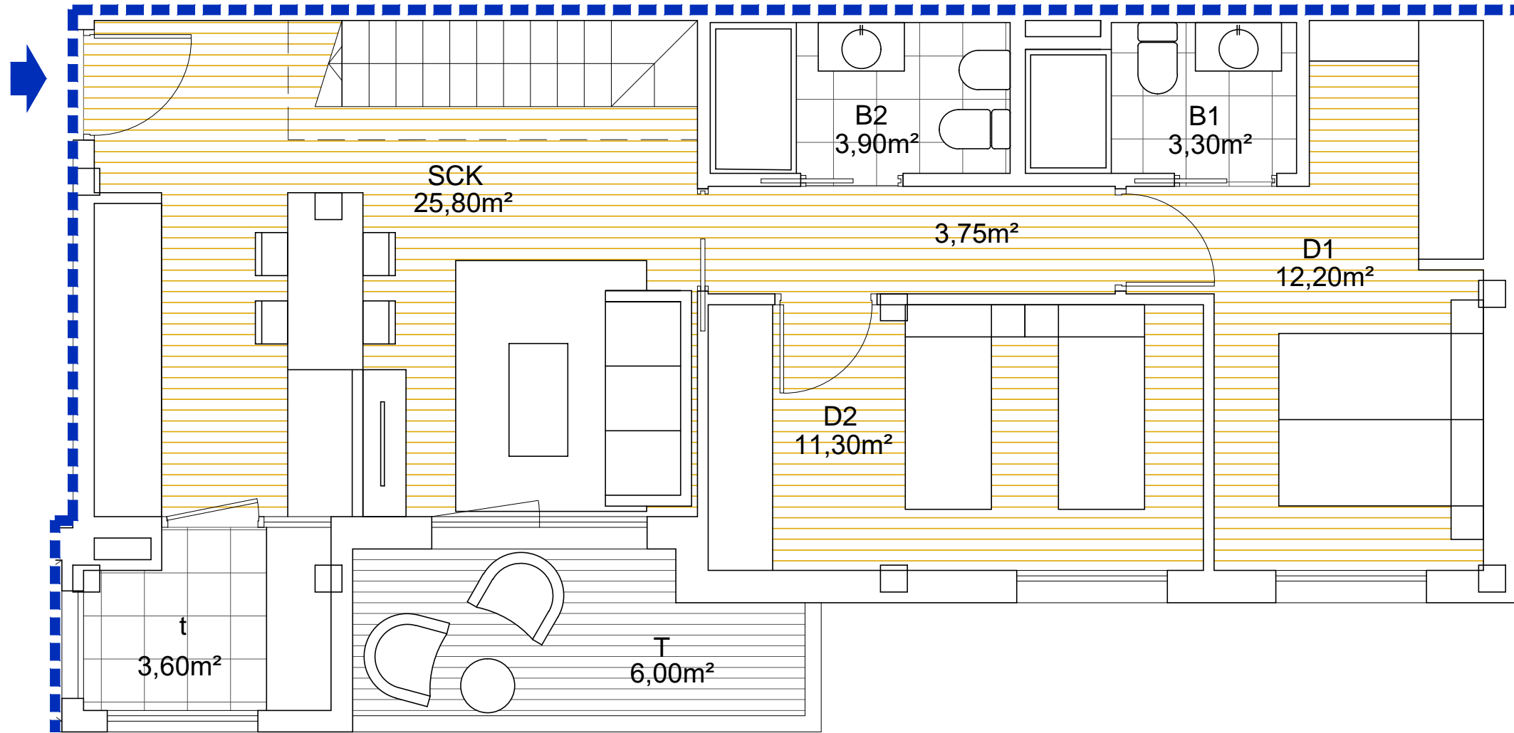
PLANTA TERCERA
