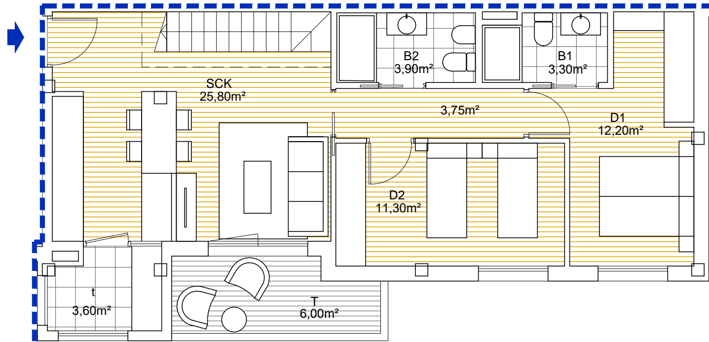
PLANTA TERCERA
