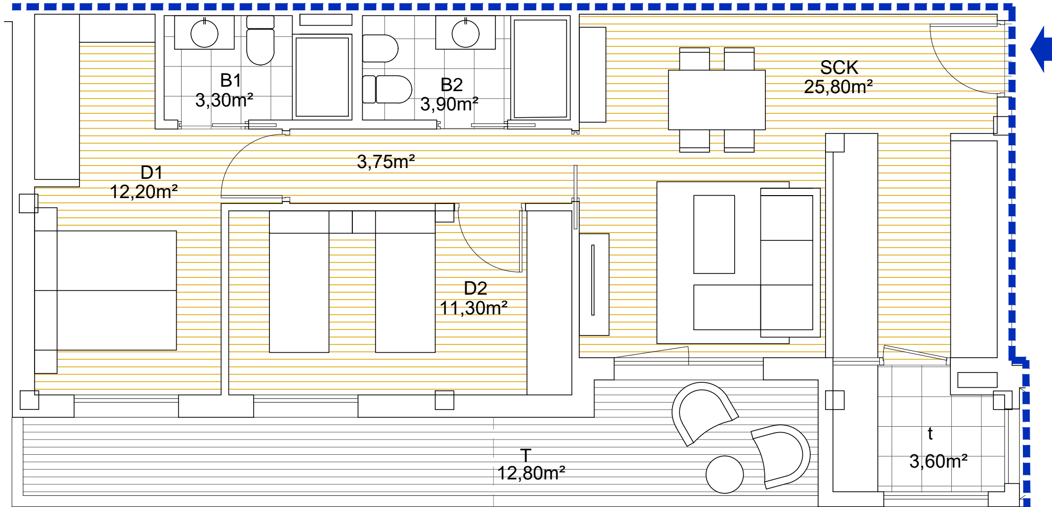
PLANTA TERCERA
