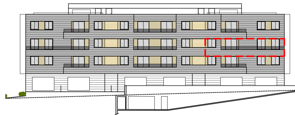
ALZADO TRASERO
