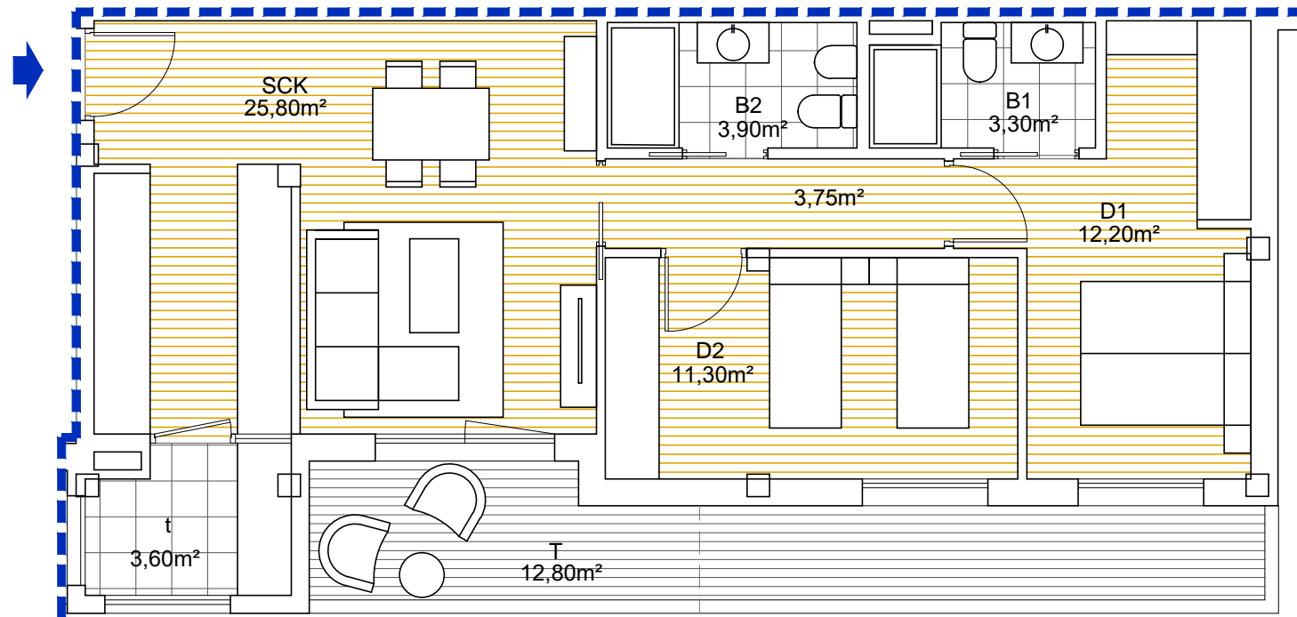
PLANTA SEGUNDA
